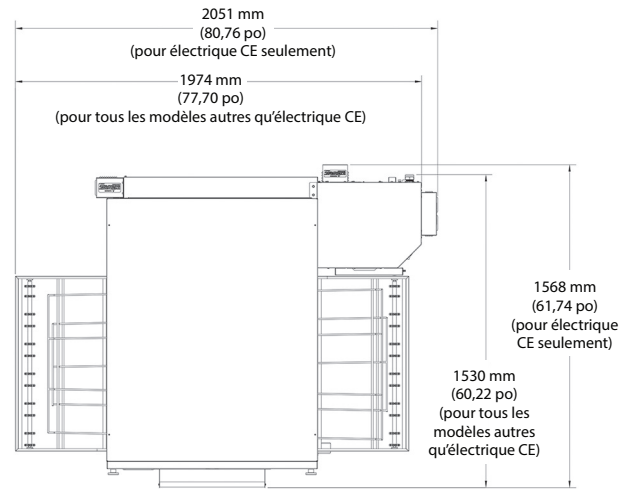
3240 Vue de dessus, toutes configurations de superposition
