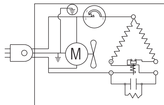
COMPRESSEUR
