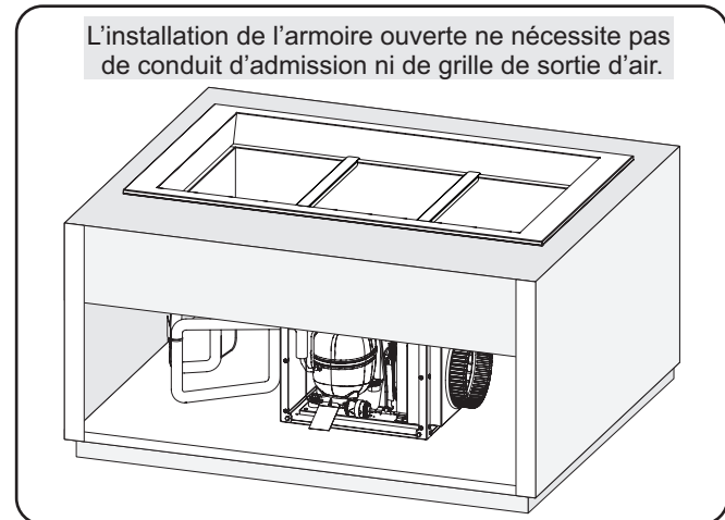
Installation de l'armoire ouverte (Modèle CWBP-3 illustré)
